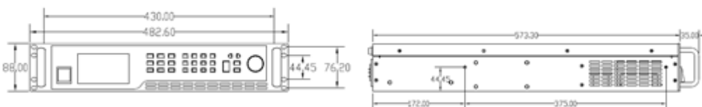
2U机型尺寸图:
